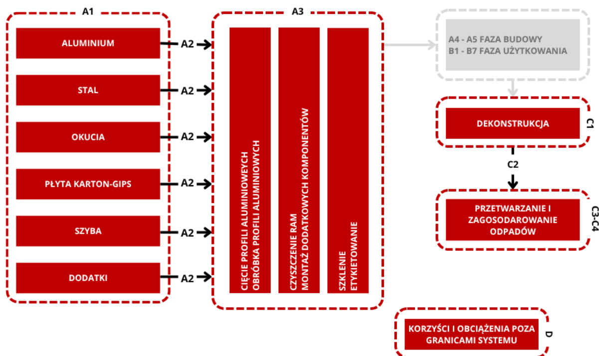
Rysunek 5.1: Granice systemu dla charakterystyki środowiskowej przeciwpożarowych drzwi aluminiowych
